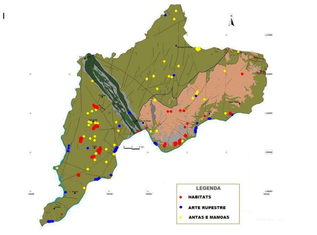
Figura 3. Distribuição global dos sítios da Pré-História Recente no concelho de Vila Velha de Ródão, sobre Carta Geológica do Concelho de Vila Velha de Ródão (seg. Carvalho et al. , 2006).
