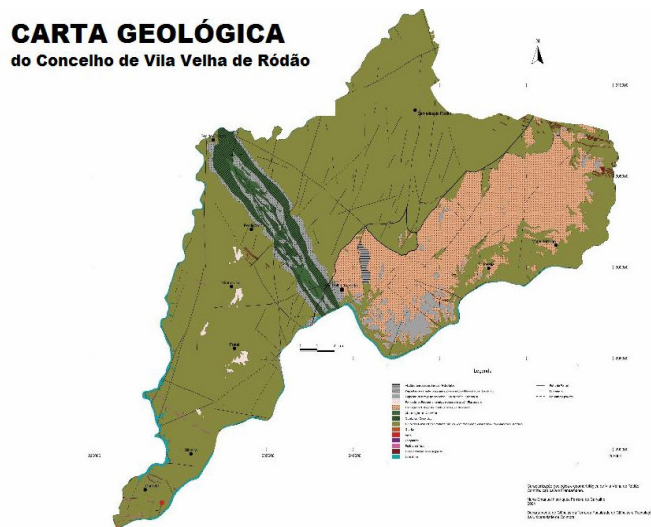
Figura 2 – Carta Geológica do Concelho de Vila Velha de Ródão (seg. Carvalho et al. , 2006).
