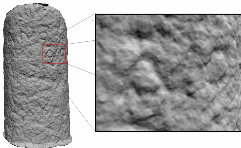
Figura 2. Vista do modelo tridimensional obtido por técnicas de fotogrametria digital.
