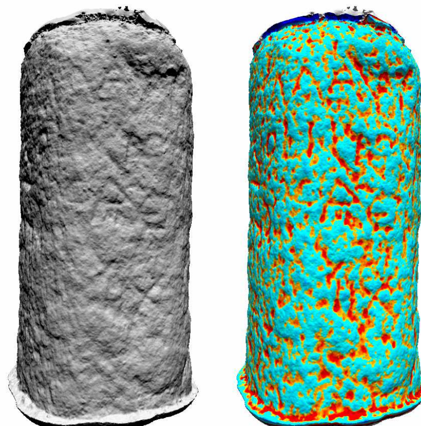
Figura 3. Vista comparativa do modelo tridimensional e do Modelo de Resíduo Morfológico do marco miliário.
