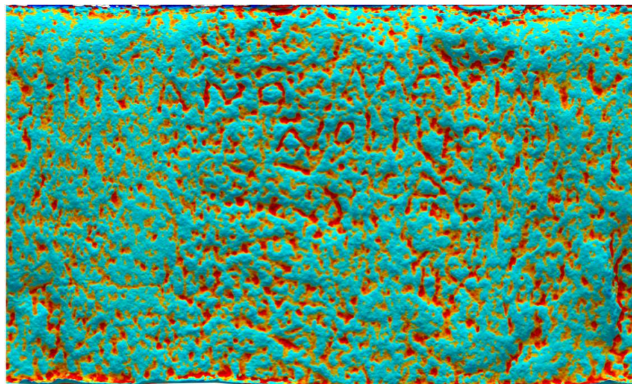
Figura 4. Imagem planificada da superfície do marco miliário com o resultado do Modelo de Resíduo Morfológico.
